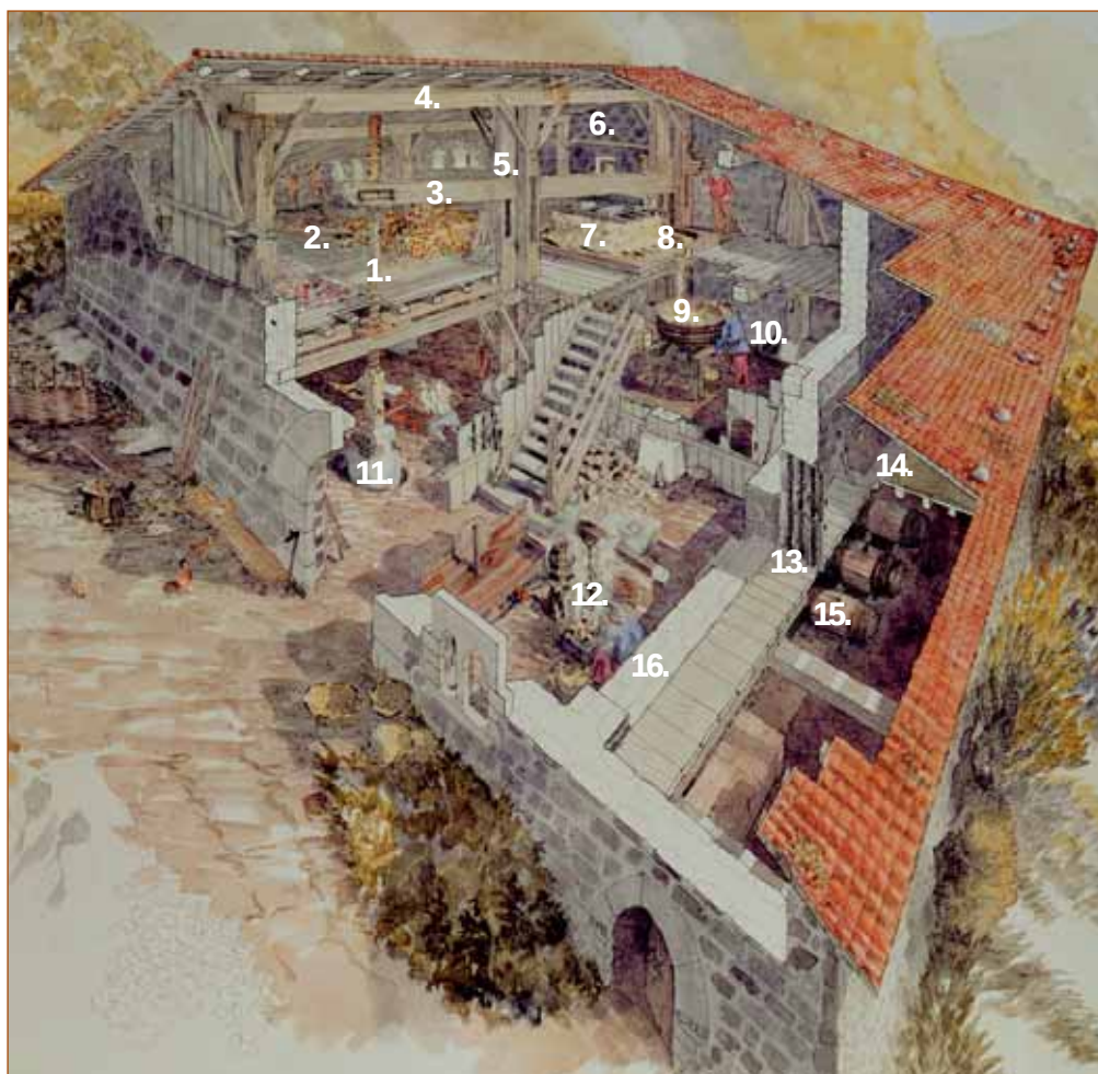
XVI. mendeko tolare baserri baten irudia. Sarobe baserrian dagoen tolarearen funtzionamendua antzekoa da. Gipuzkoako Foru Aldundiko Kultura Sailak utzitako marrazkia. Gidoia: Alberto Santana. Marrazkia: Ramón Urain.
